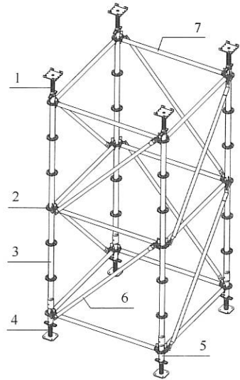
图2 承插型盘扣式钢管 脚手架示意二
